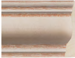
Référence: RMG-1616/6074 Noir mat côté gratté Dim.: 68mm x 38mm Feuillure: 10mm x 8mm Finition: Renversé creux
